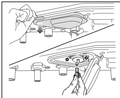
fig. 13 Instellen uitstroomhoeveelheid warm tapwater
