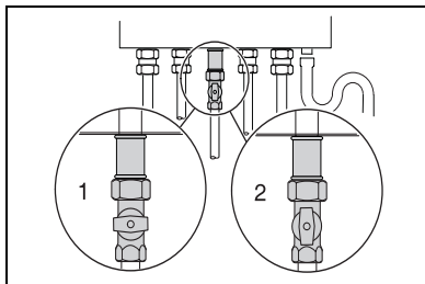
fig. 15 Gaskraan
