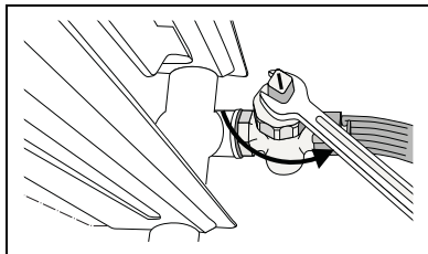
fig. 16 Aftappen van de cv-installatie
